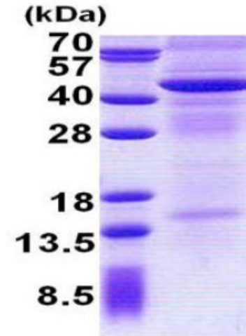
15% SDS-PAGE (3µg)
